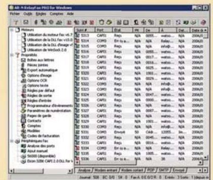
Interface d'administration principale
